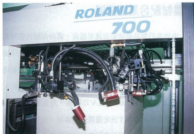
安裝在飛達上的靜電消除器，有利於印刷薄膜材料
